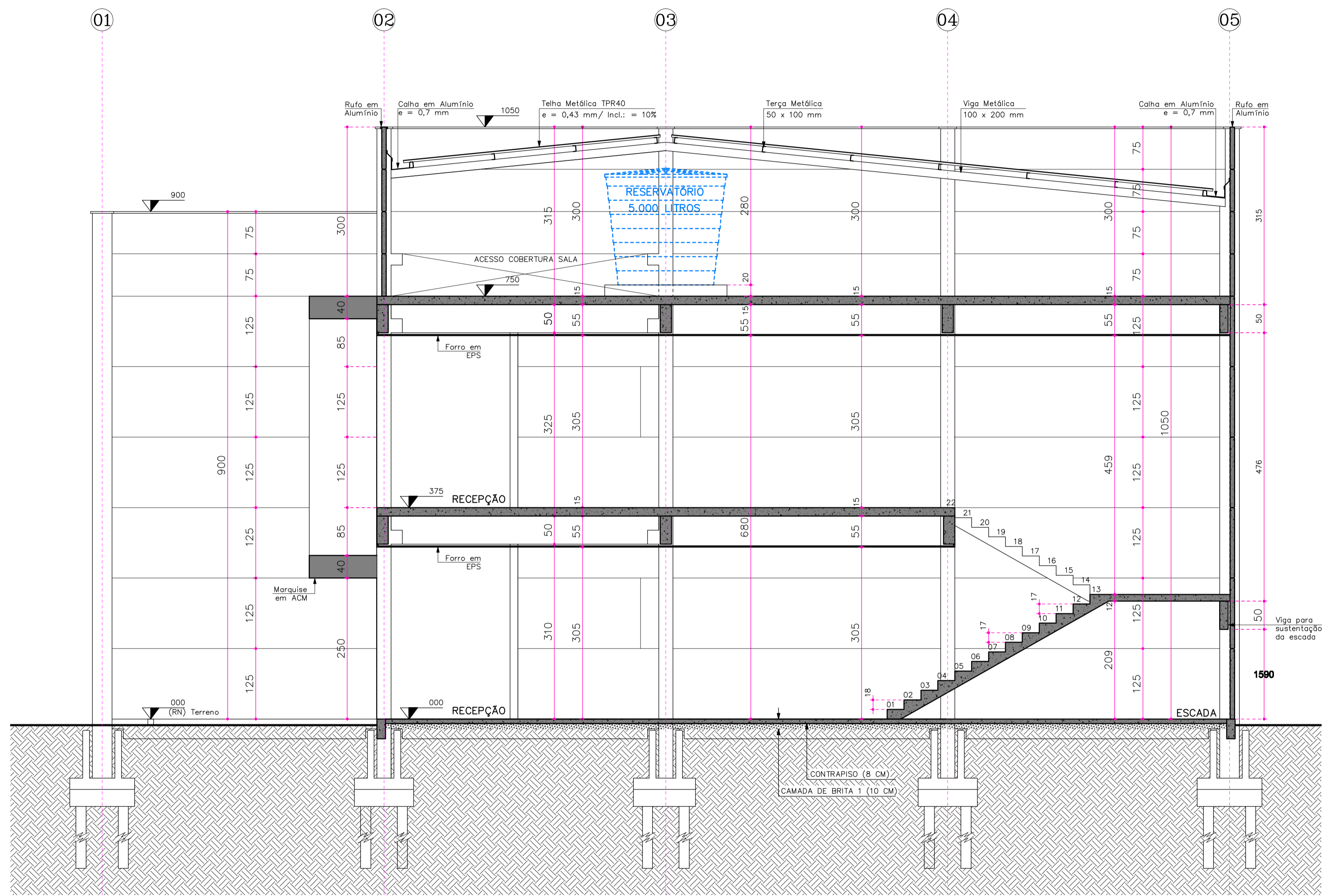
CORTE - BB' -
