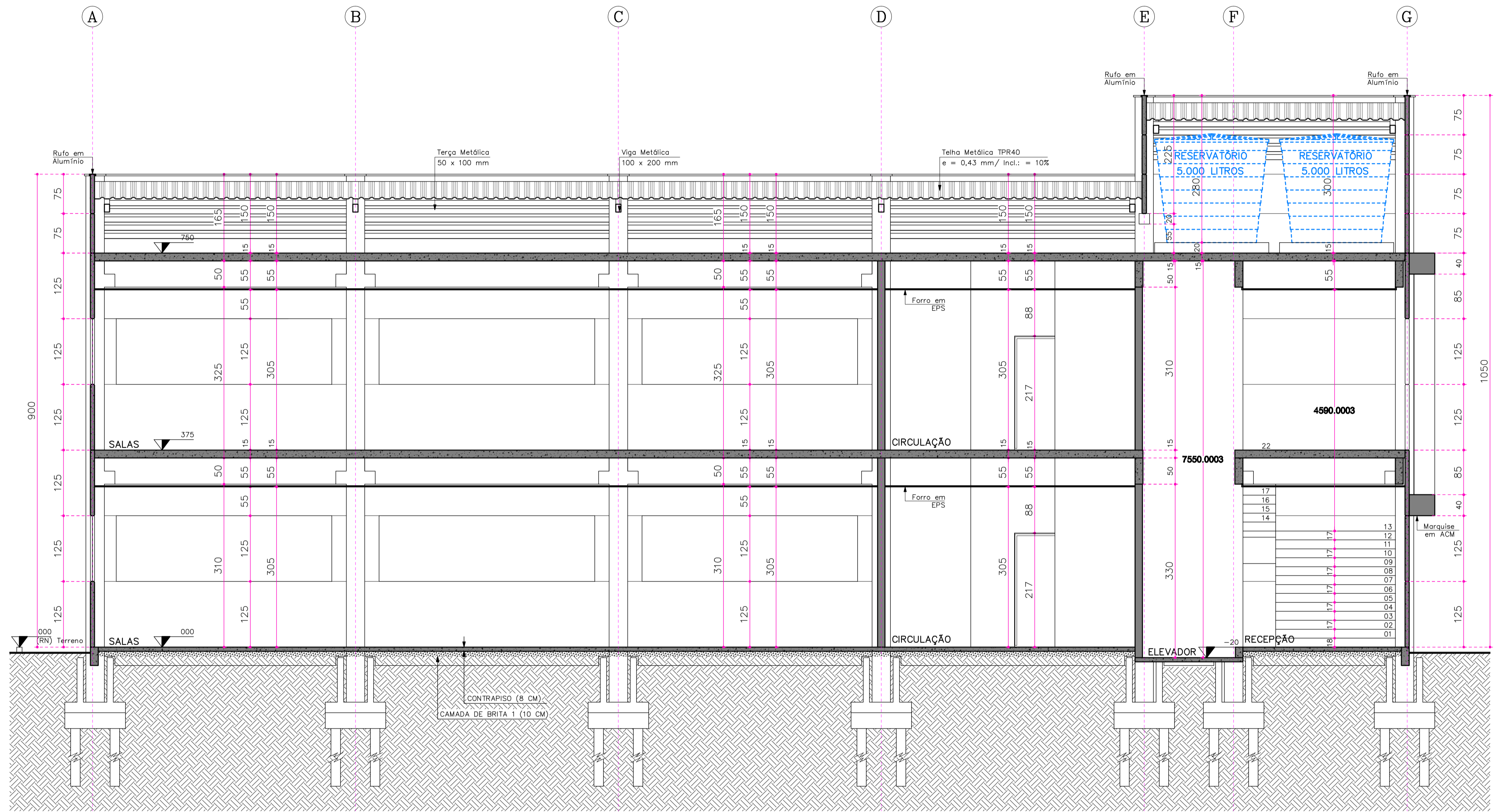
CORTE - CC' -
