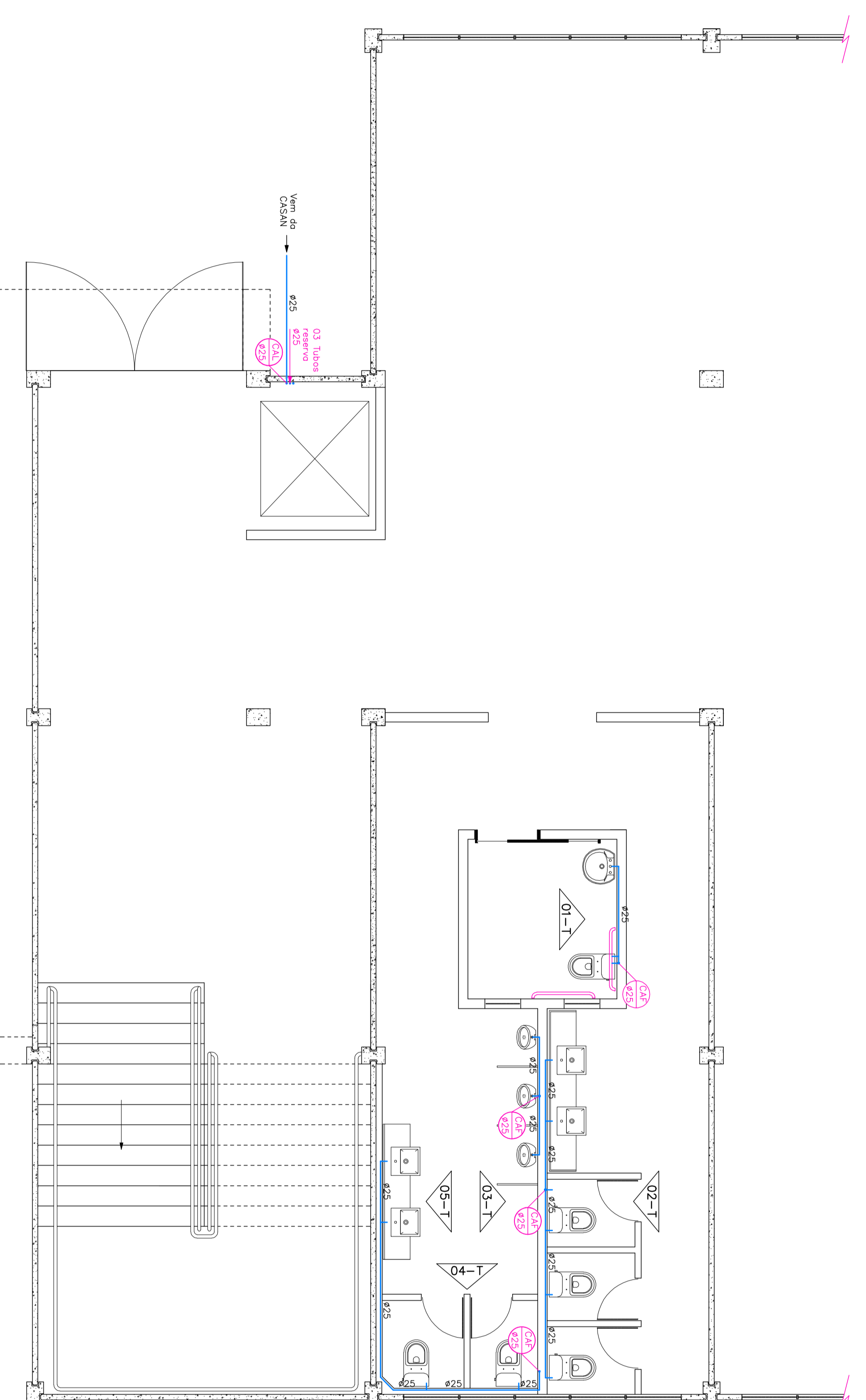
PLANTA DO SISTEMA DE DISTRIBUIÇÃO DE ÁGUA – TERREO (HIDRÁULICO)
