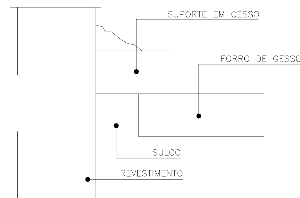
Detalhe - Junta de Dilatação Sem Escala
