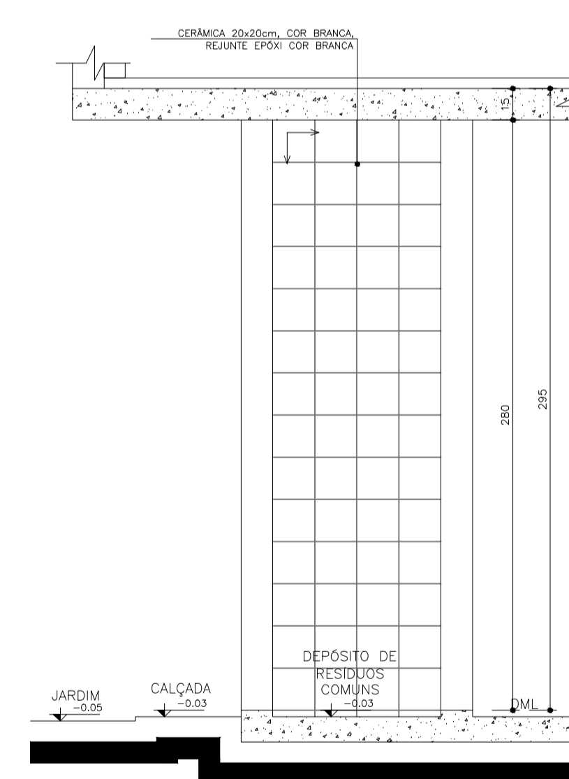
07 Seção BB' ABRIGO DE RESÍDUOS COMUNS Esc.: 1:25
