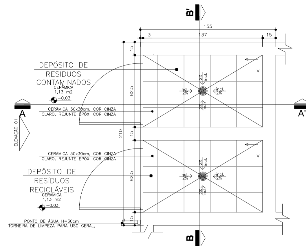
01 Planta Baixa ABRIGO DE RESÍDUOS RECICLÁVEIS E CONTAMINADOS Esc.: 1:25
