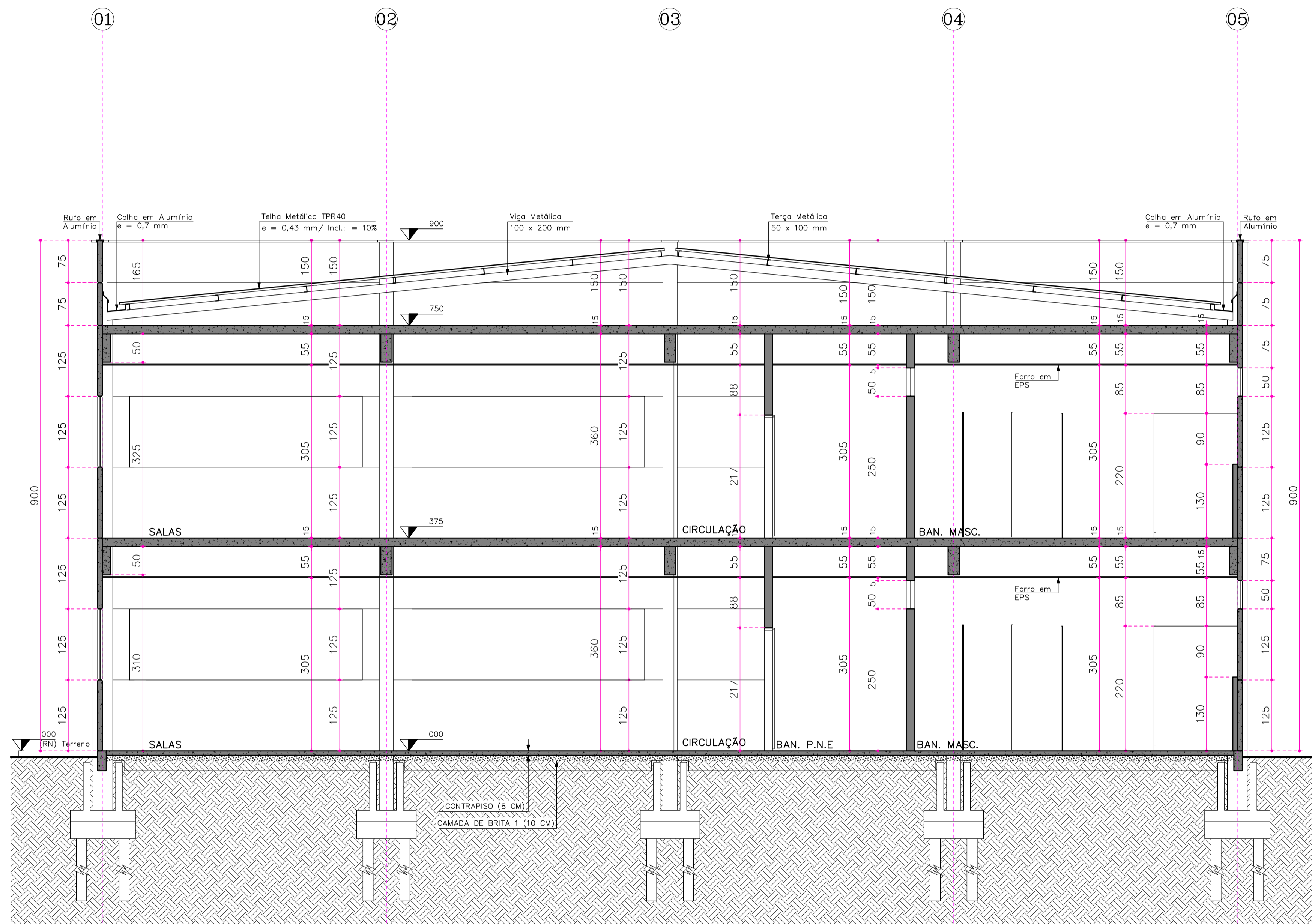
CORTE - AA' -
