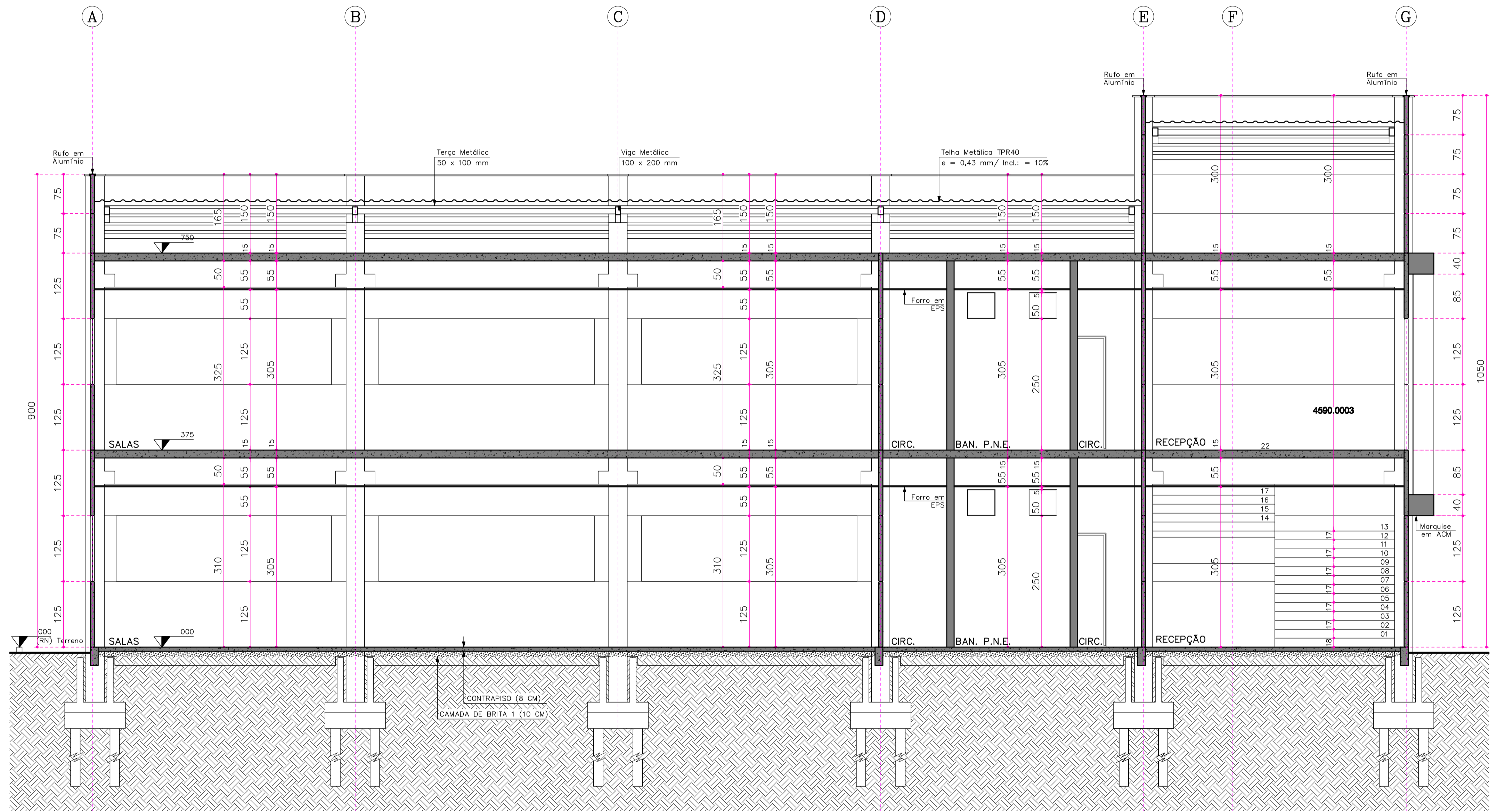
CORTE - DD' -
