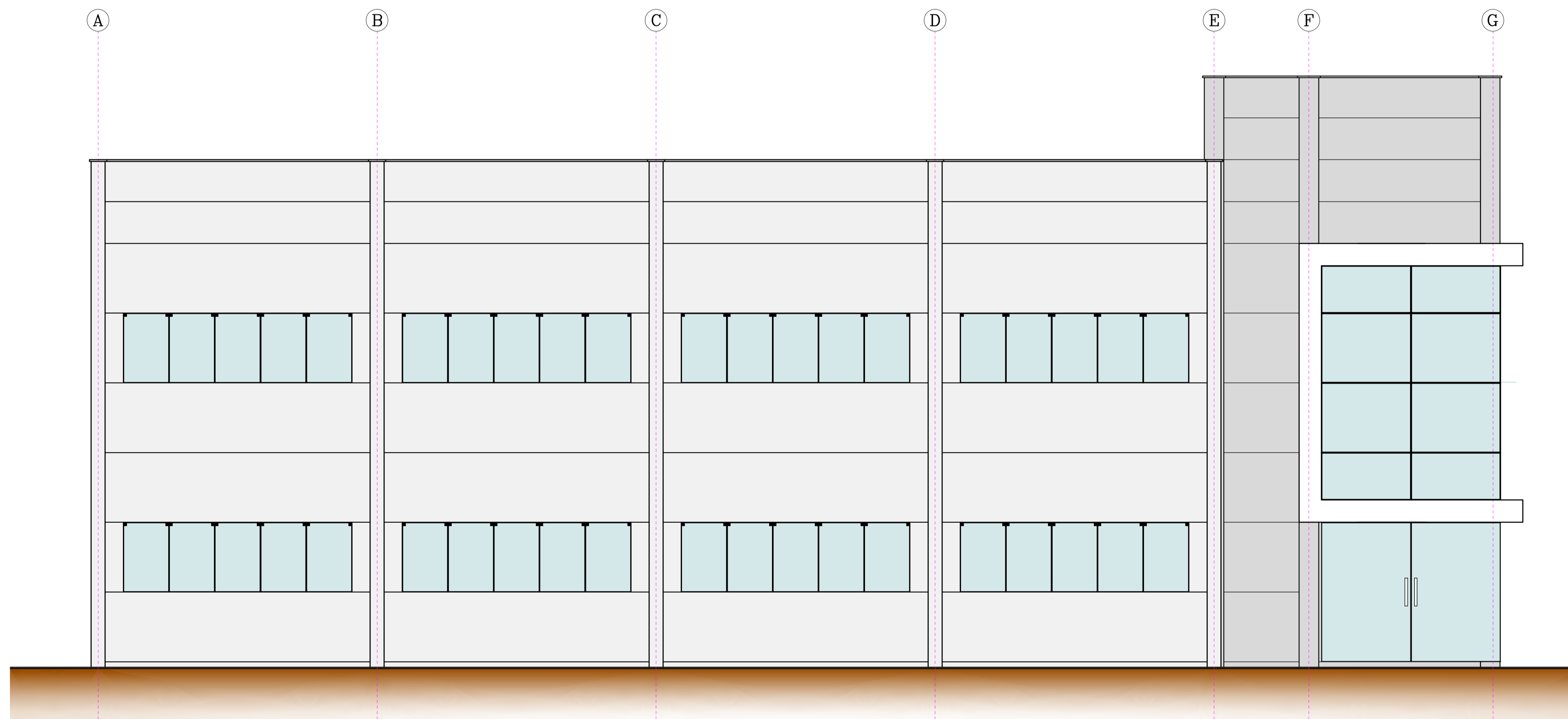
ELEVAÇÃO - 03
