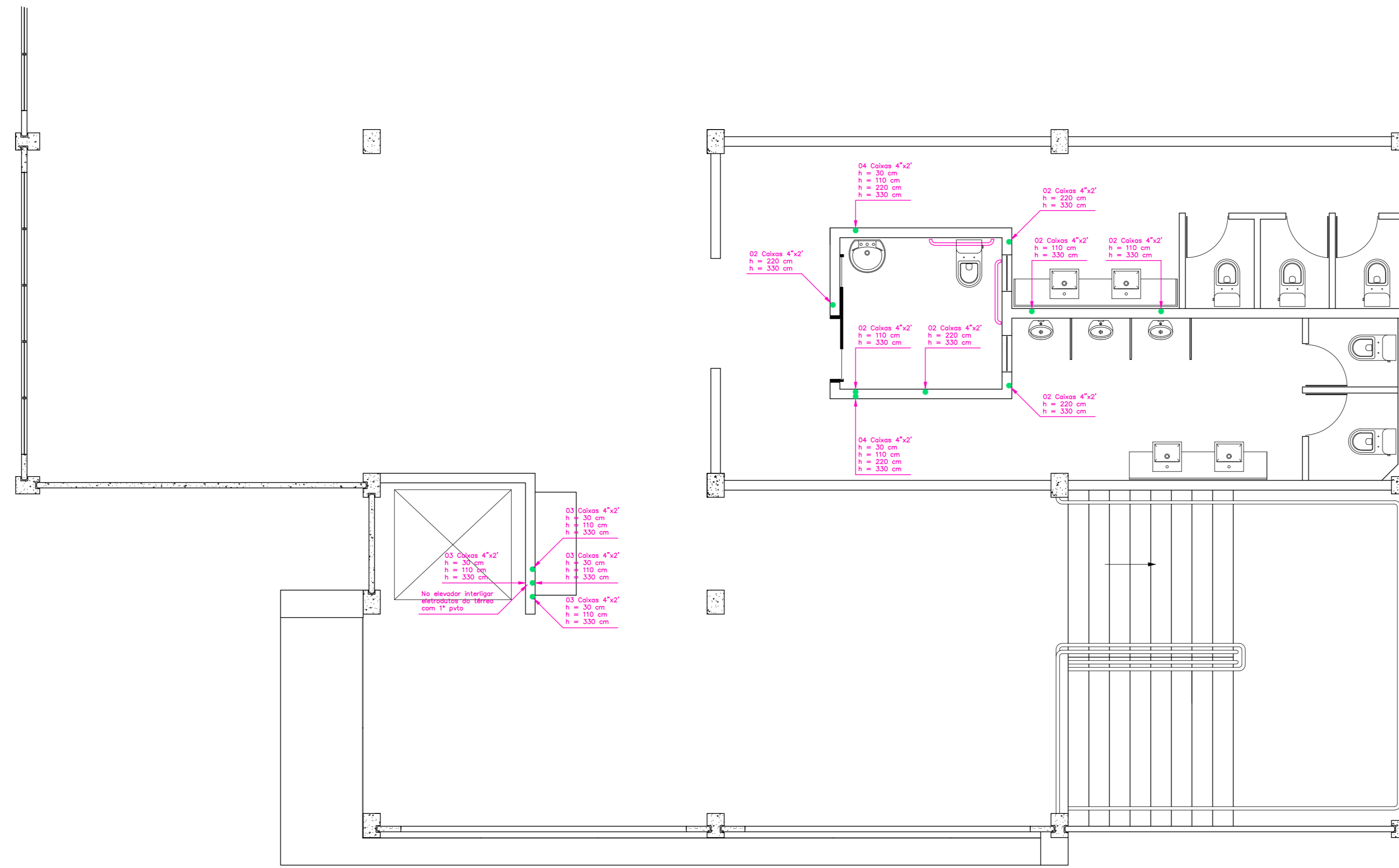
DIAGRAMA EM PLANTA (ELÉTRICO) - 1º PVT0
