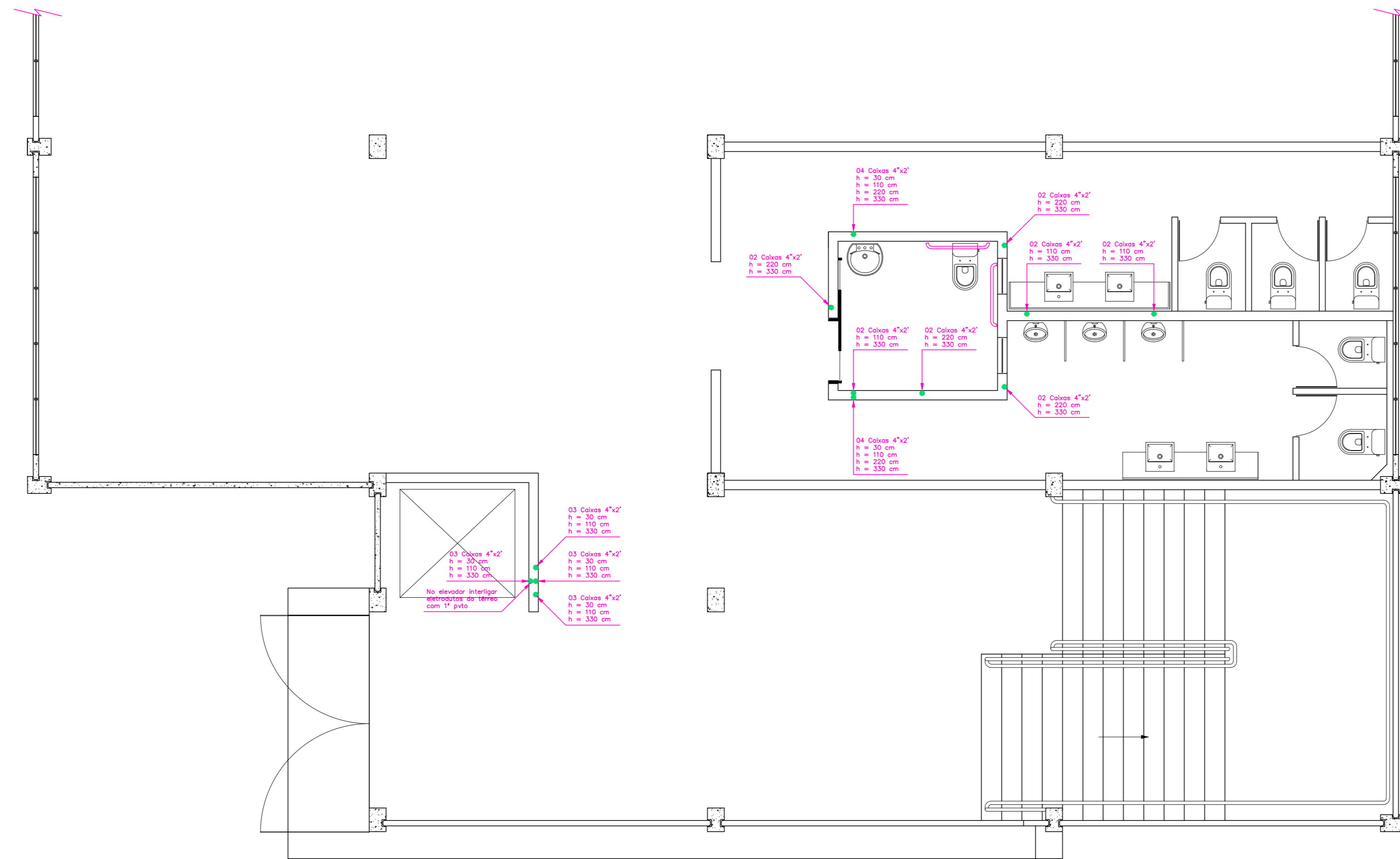
DIAGRAMA EM PLANTA (ELÉTRICO) - TÉRREO
