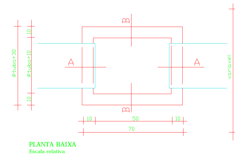
PLANTA BAIXA Escala relativa
